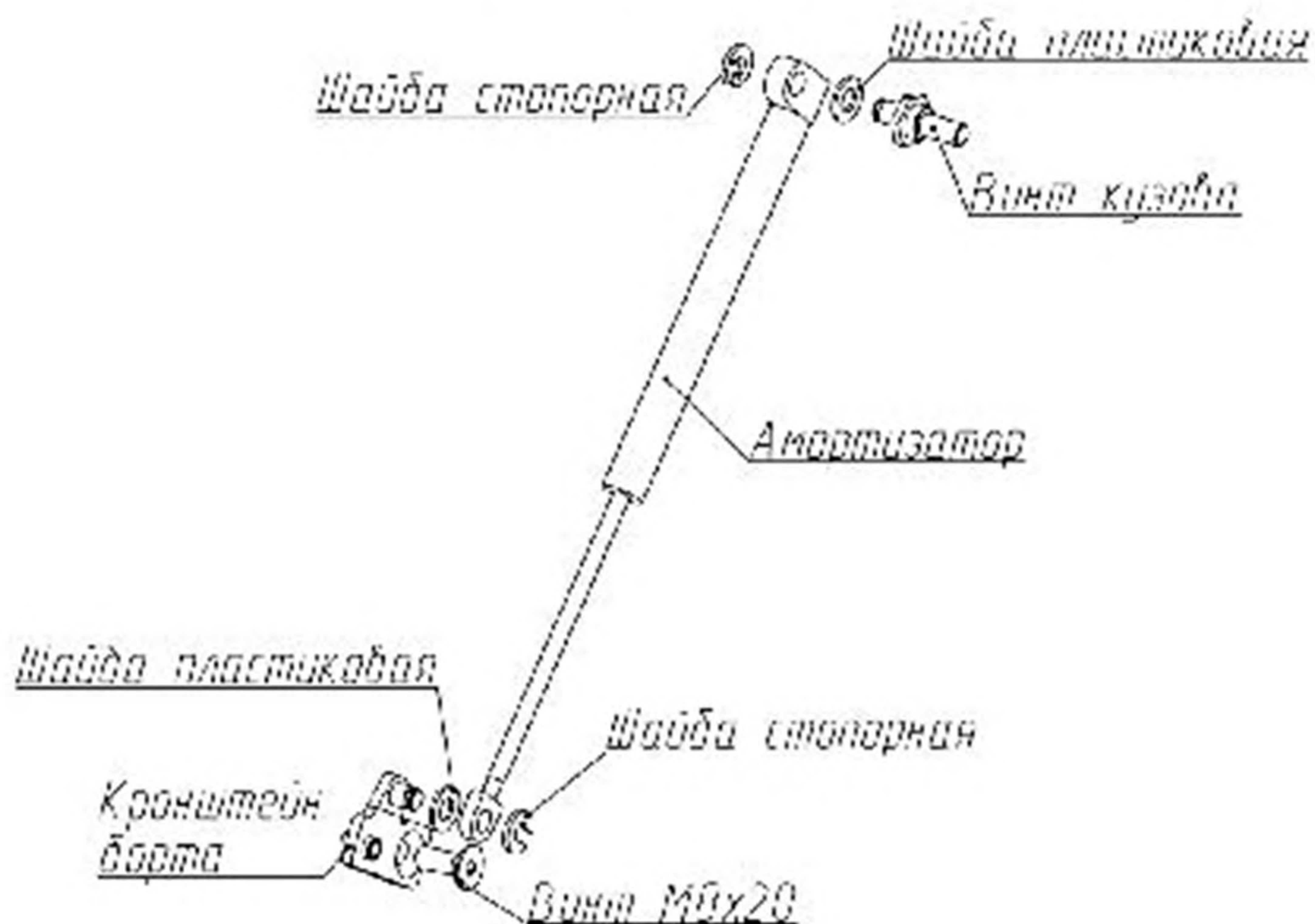
Схема установки
