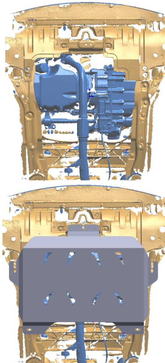
Защита ДВС
